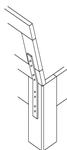
Eisenbeschlag für schräge Kopfteile
